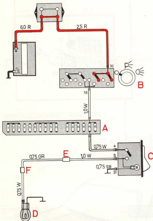
Commutateur d'éclairage actionné, interrupteur d'antibrouillard AR non actionné
