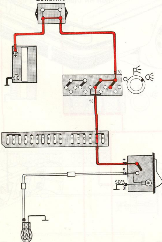
Commutateur d'éclairage actionné, interrupteur d'antibrouillard AR non actionné
