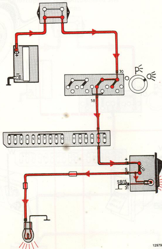
Commutateur d'éclairage et interrupteur d'antibrouillard AR actionnés
