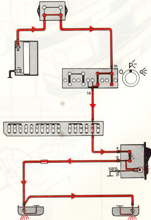
Commutateur d'éclairage et interrupteur d'antibrouillard AR actionnés
