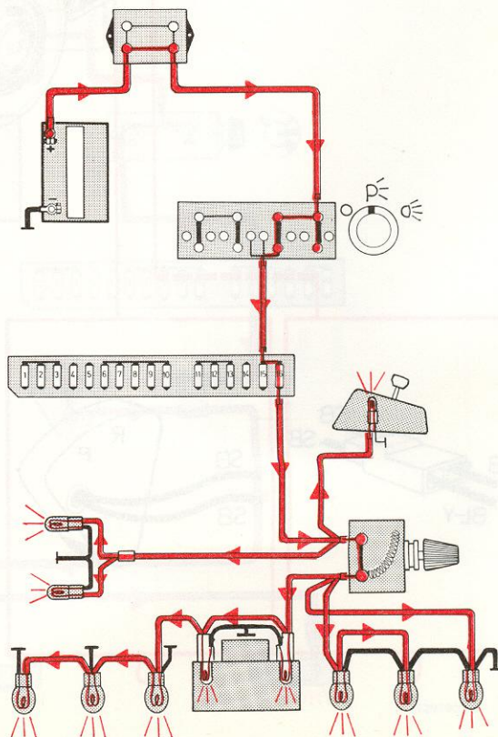
Commutateur d'éclairage actionné Rhéostat hors circuit
