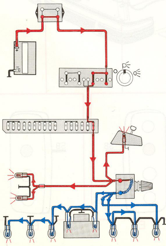
Commutateur d'éclairage actionné Rhéostat entièrement en circuit
