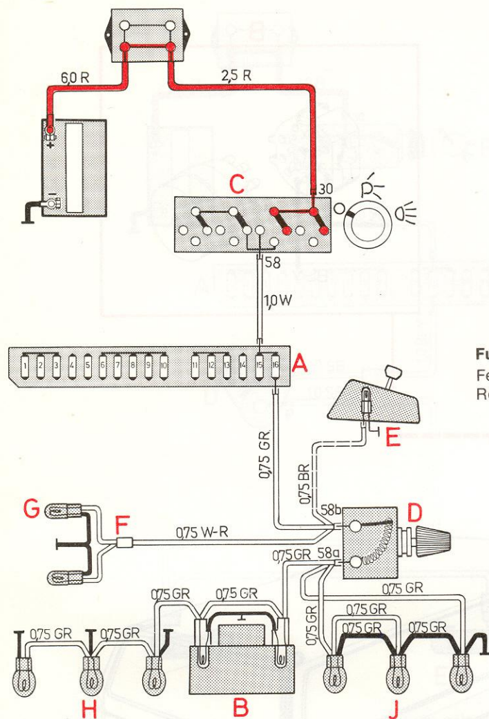
Commutateur d'éclairage actionné Rhéostat entièrement en circuit
