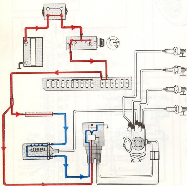
Unité de commande laissant passer le courant, charge de la bobine
