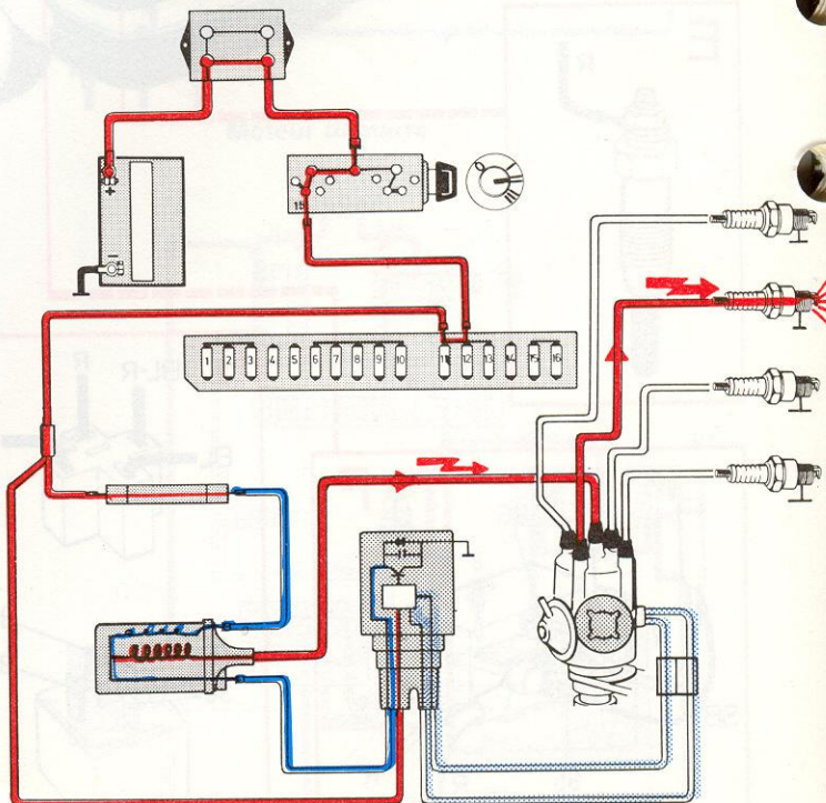
Unité de commande coupant le courant, décharge de la bobine
