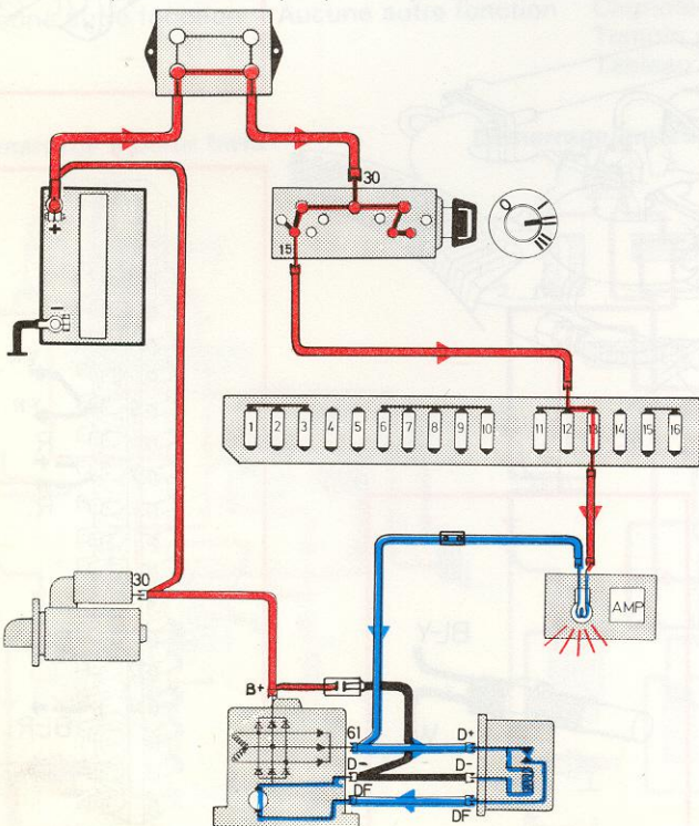
Contact mis (moteur au repos)
