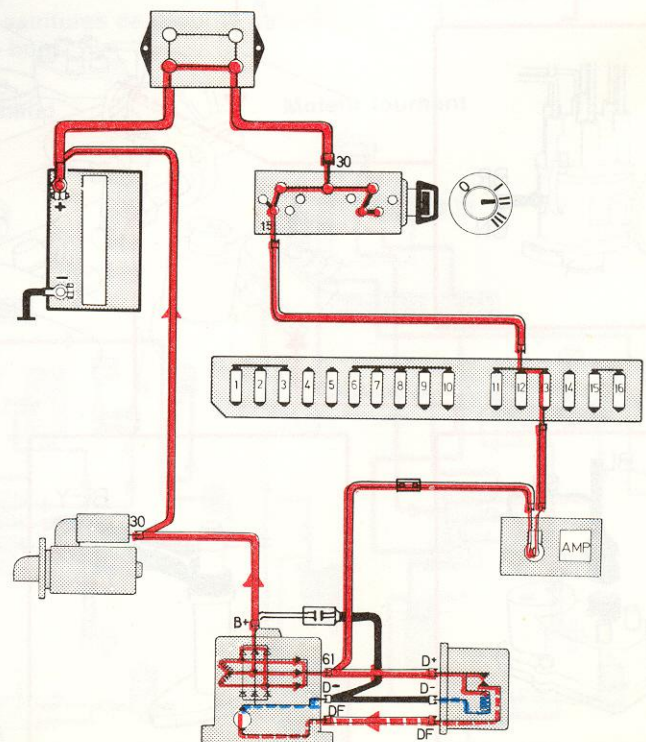
Charge par l'alternateur
