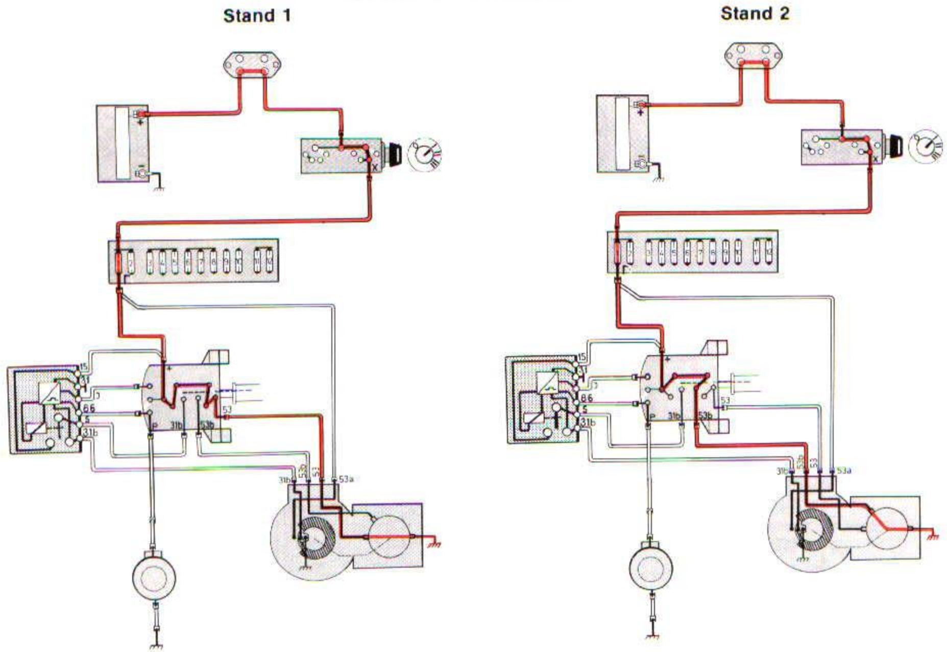
Wisserintervalrelais ingeschakeld
