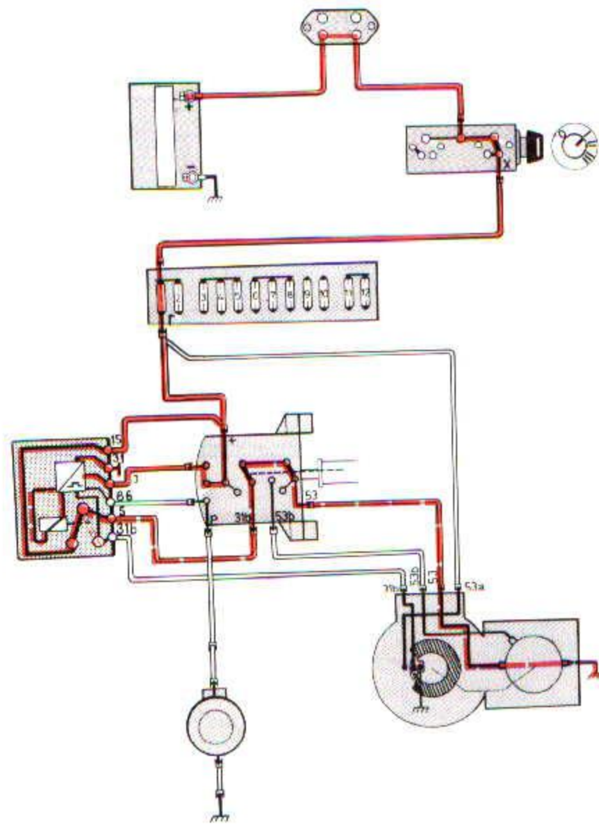
Wisserintervalrelais ingeschakeld
