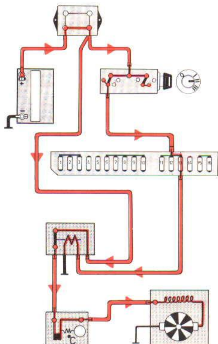
Contact aan, schakelaar thermostaat aan
