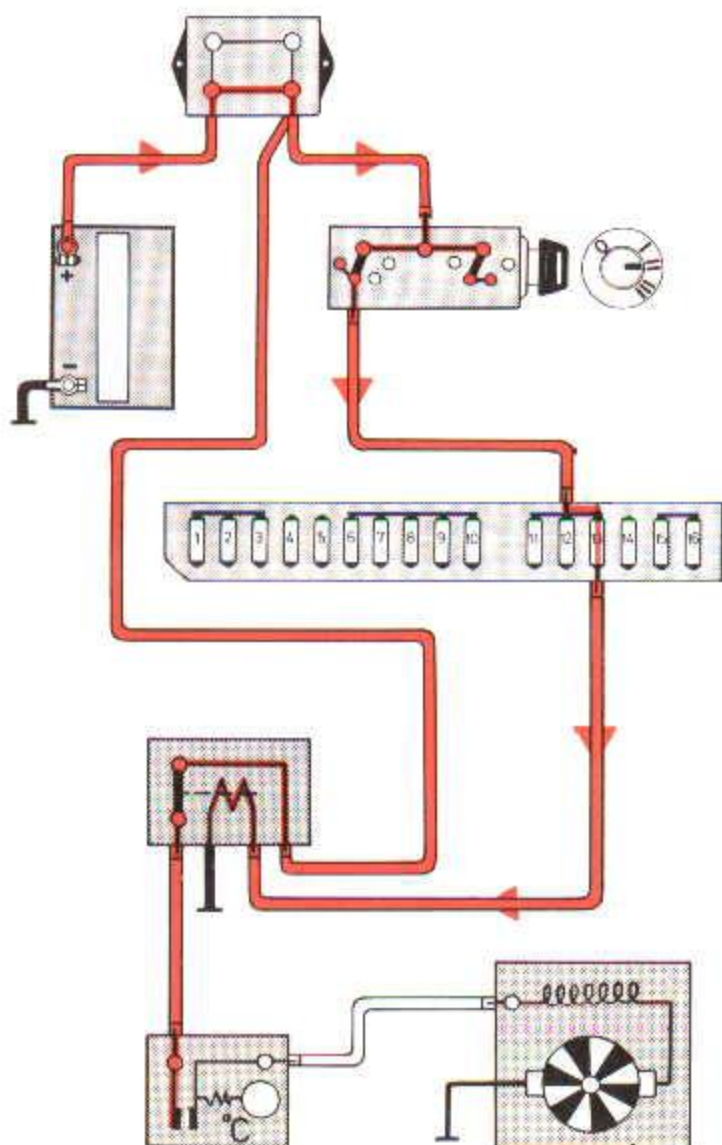
Contact aan, schakelaar thermostaat uit
