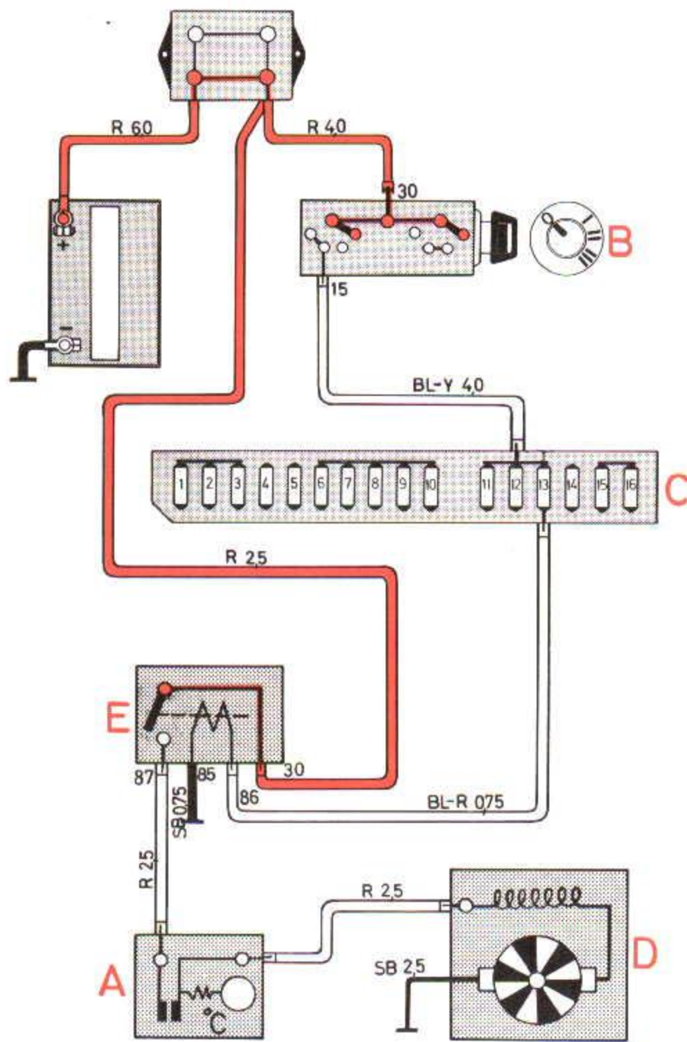
Contact aan, schakelaar thermostaat uit
