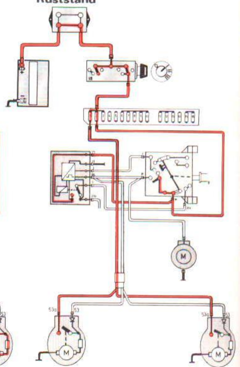
Ruststand
