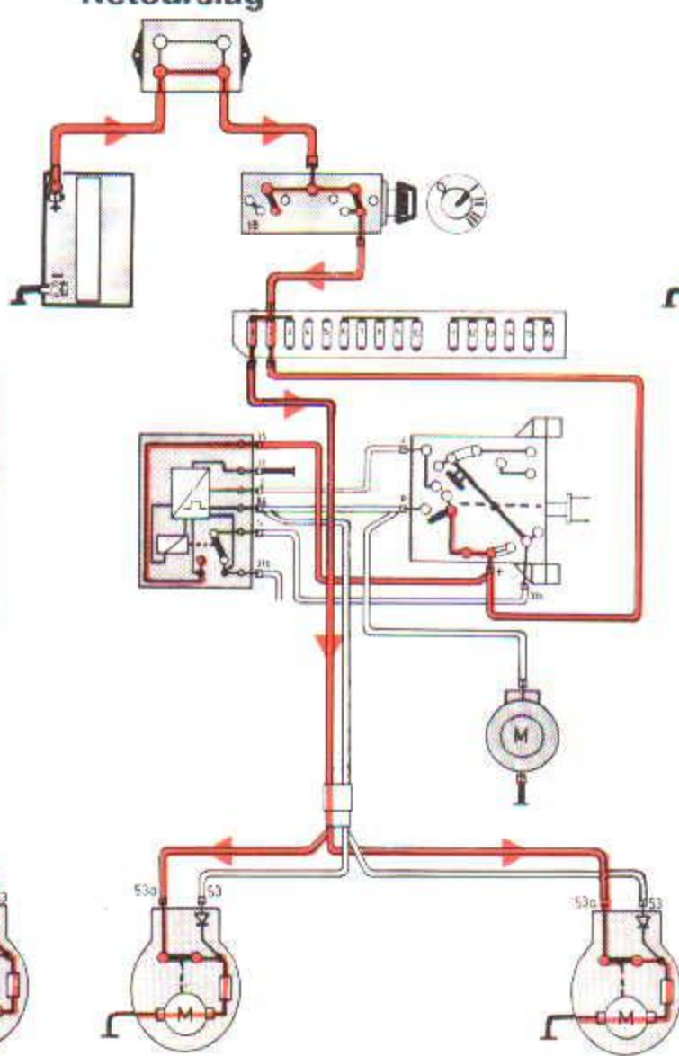
Retourslag
